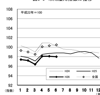
図3-5 常用雇用指数の推移
