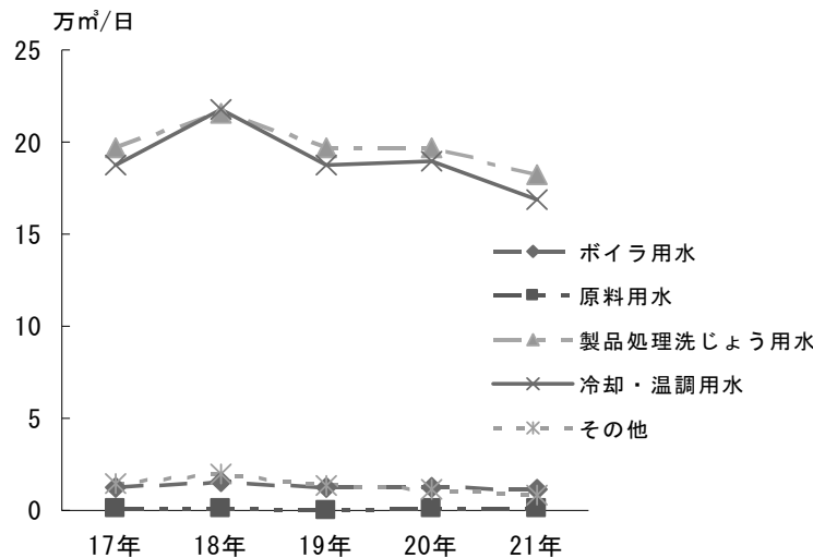
図12-7 用途別用水量の推移
